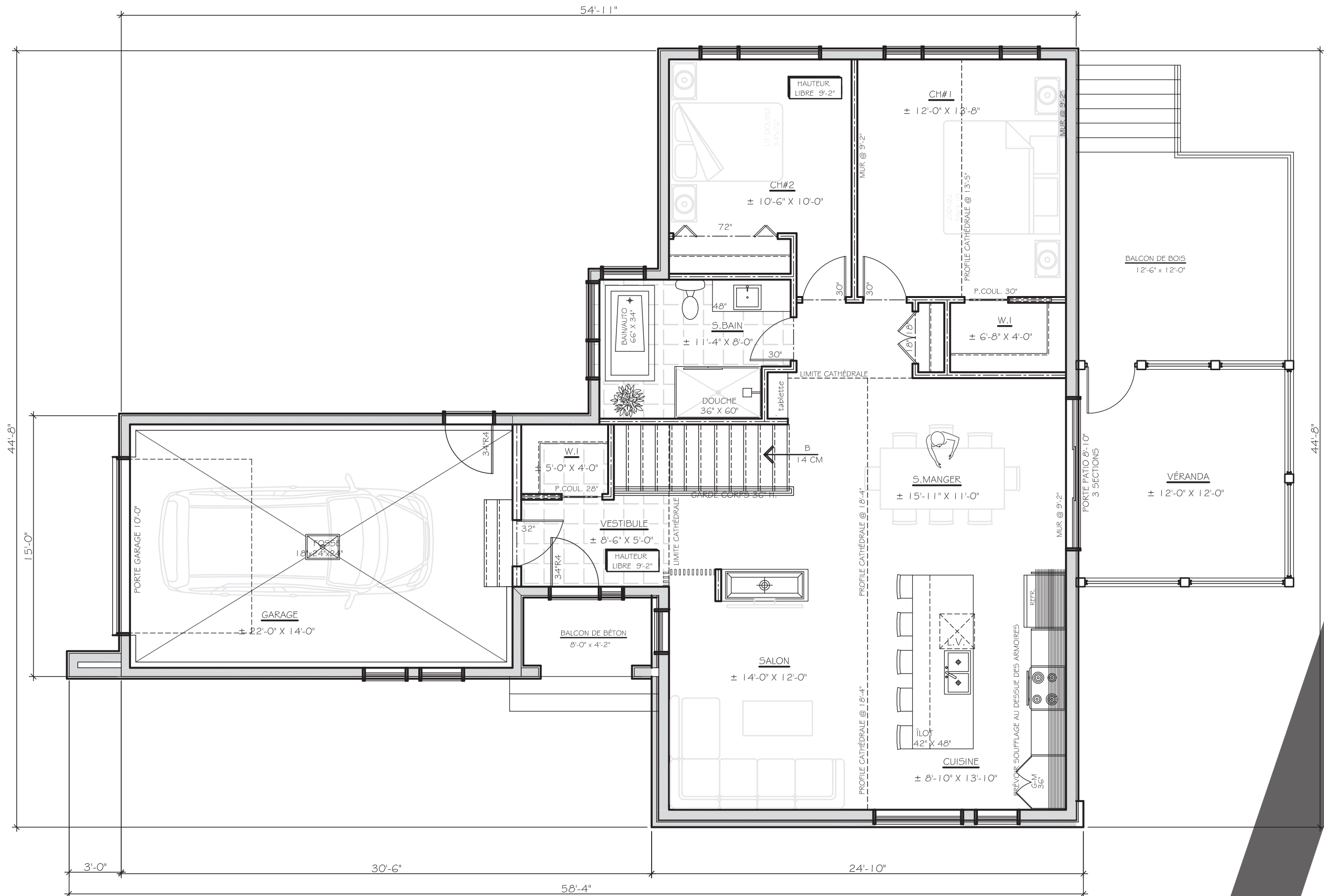
PLAN DU REZ-DE-CHAUSSÉE SUPERFICIE RDC: 1132 PI.CA SUPERFICIE GARAGE: 339 PI.CA
