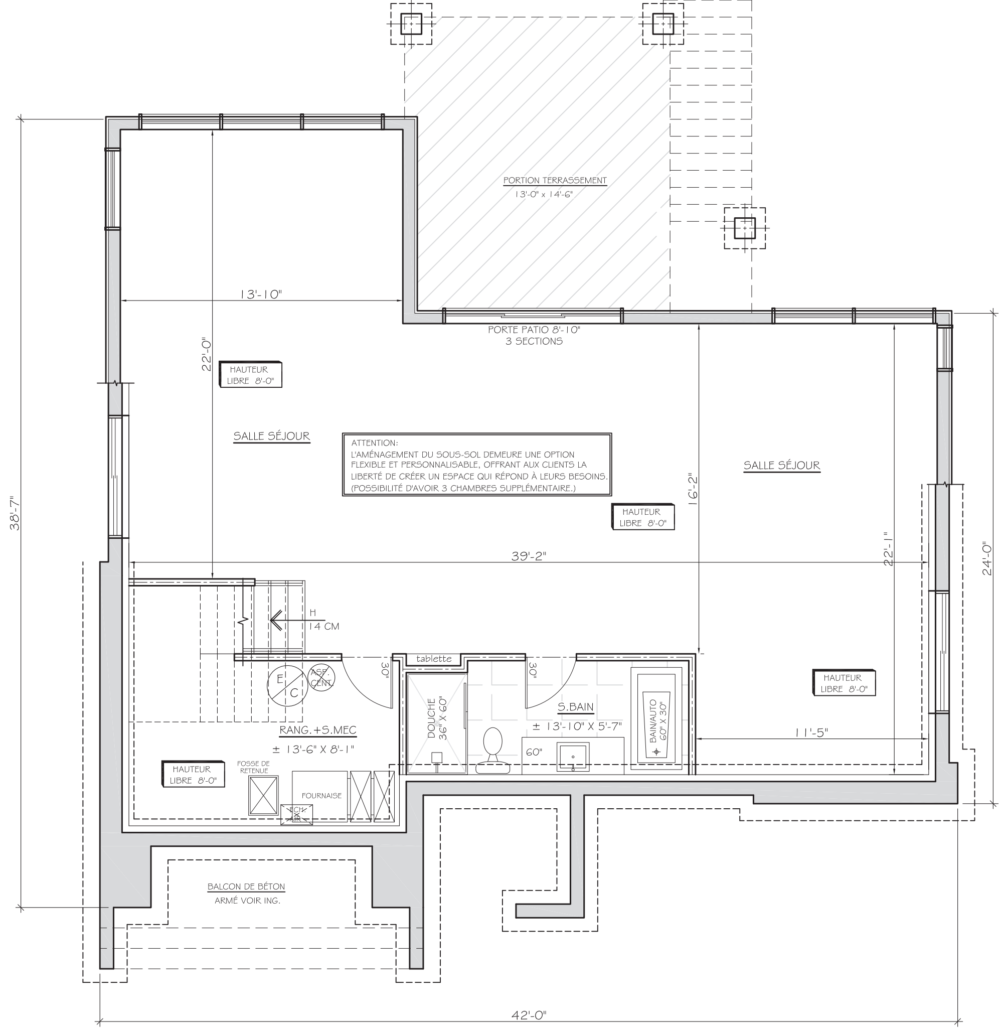
PLAN DE FONDATION
